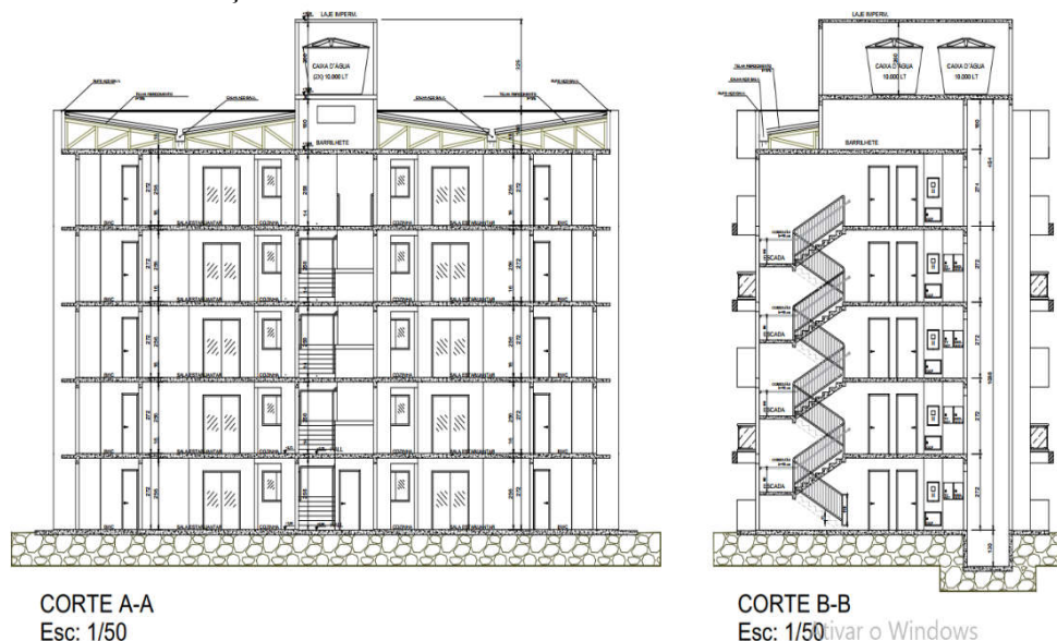
Figura 3: Cortes da edificação.
